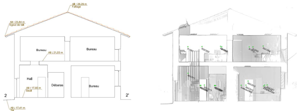
Relevé d'intérieur et coupes réalisés sur la Commune d'Orthevielle (40)
